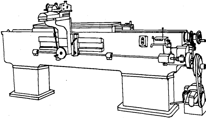
图1 长刻线机
