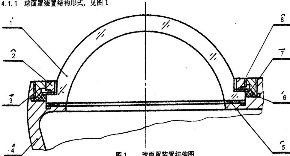
图1 球面罩装置结构图
