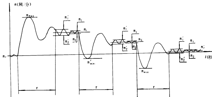
图 1 转速调节过渡过程曲线
