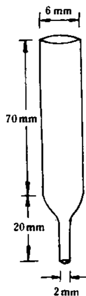
图 1 玻璃吸附管
