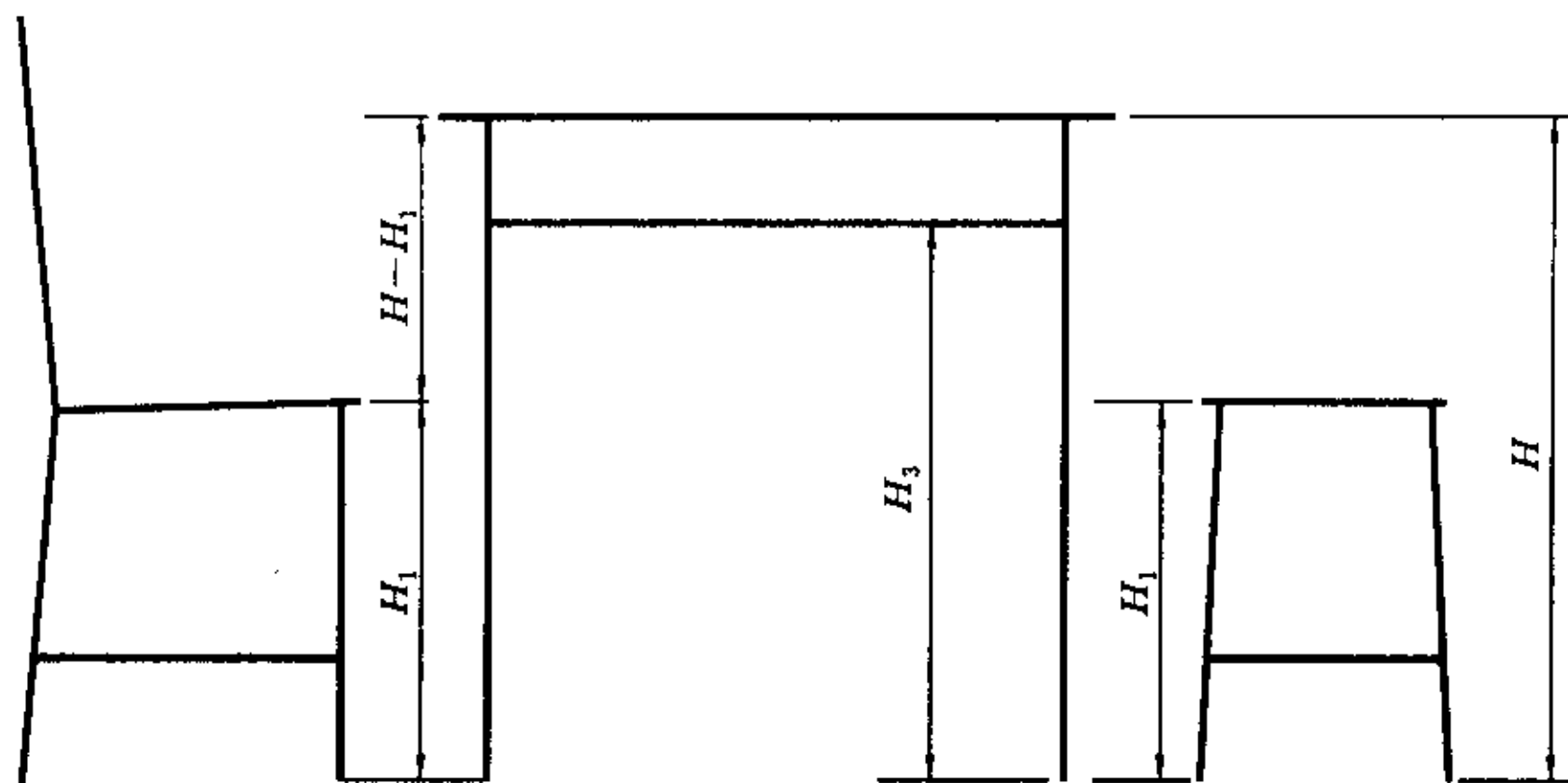
图 1 桌面高、座高、配合高差示意图
