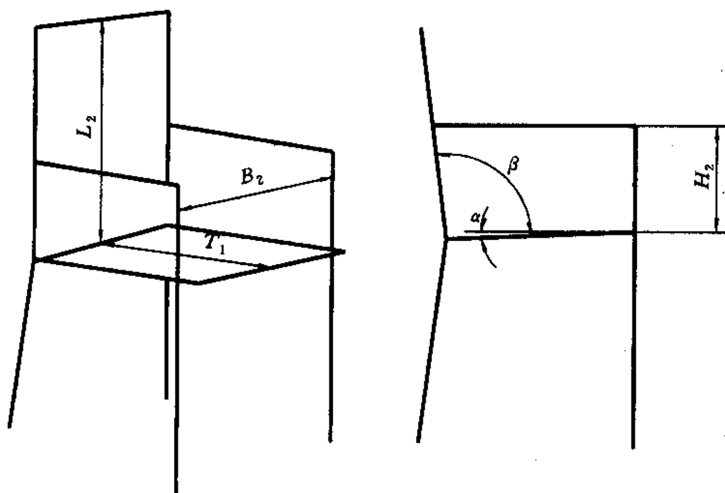
图 2 扶手椅尺寸示意图
