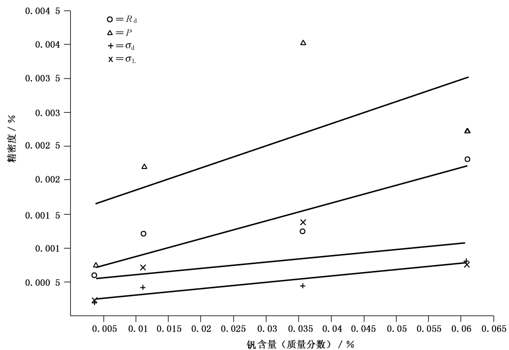
图 C.1 精密度对钒含量 X 的最小二乘法拟合图(方法 1)
