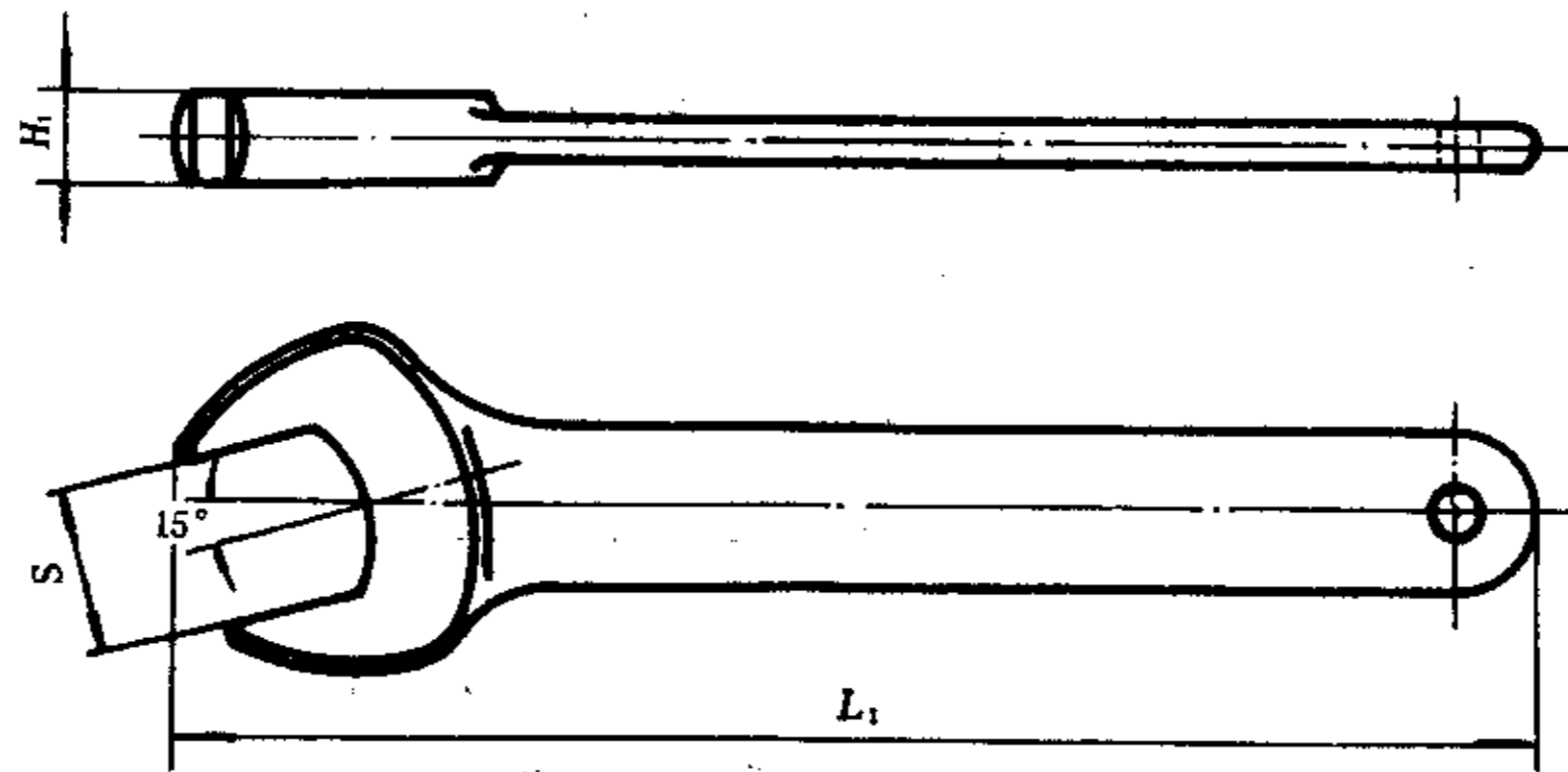
图 2 单头呆扳手
