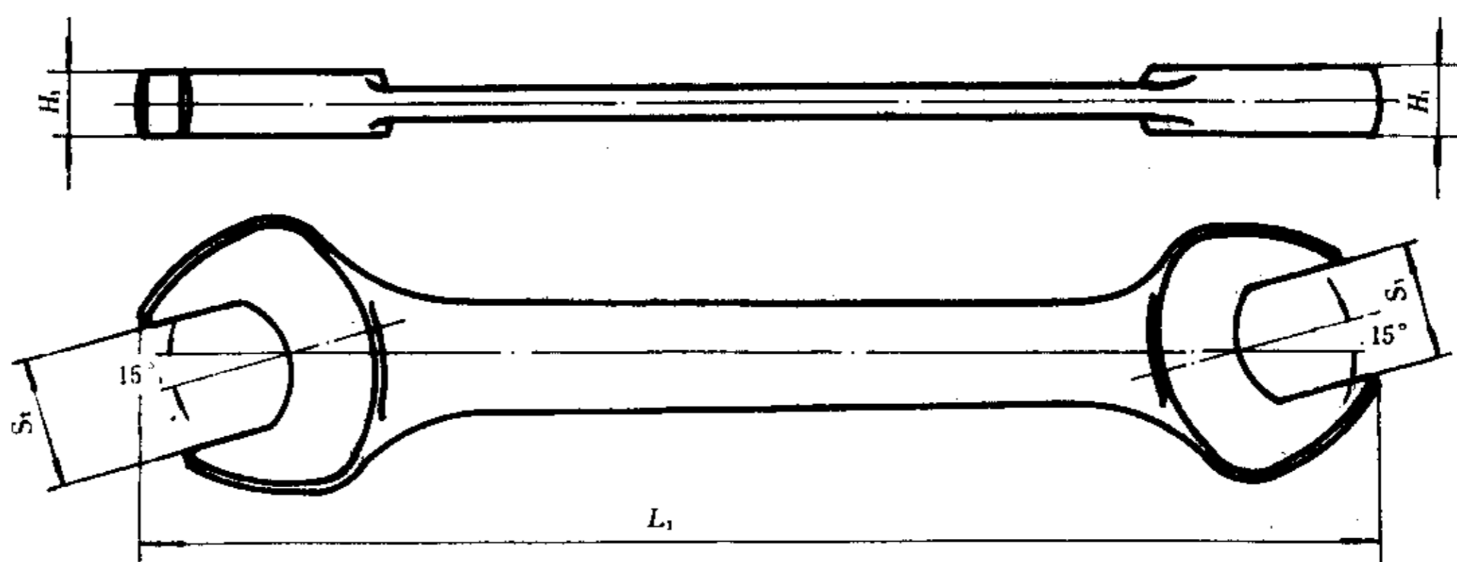
图 1 双头呆扳手
