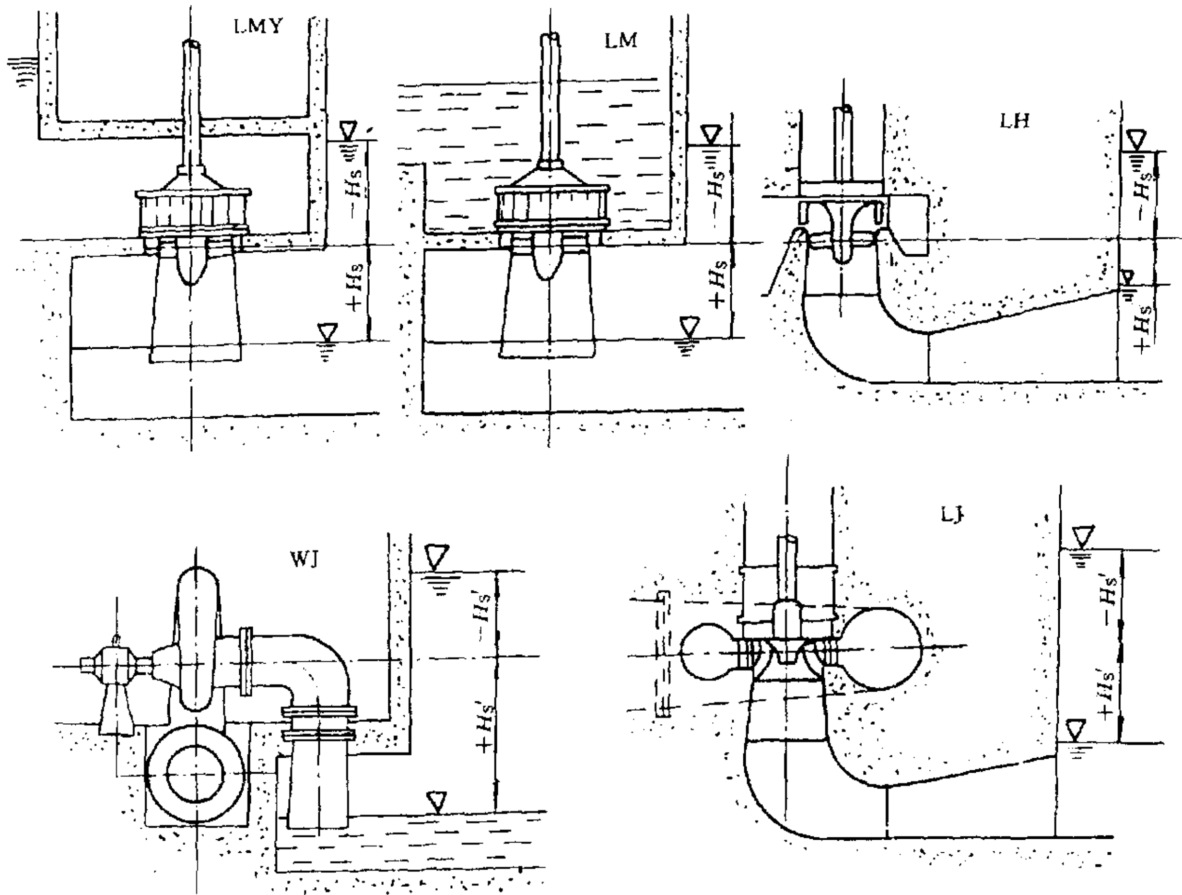
图 1 轴流式、混流式水轮机装置型式
