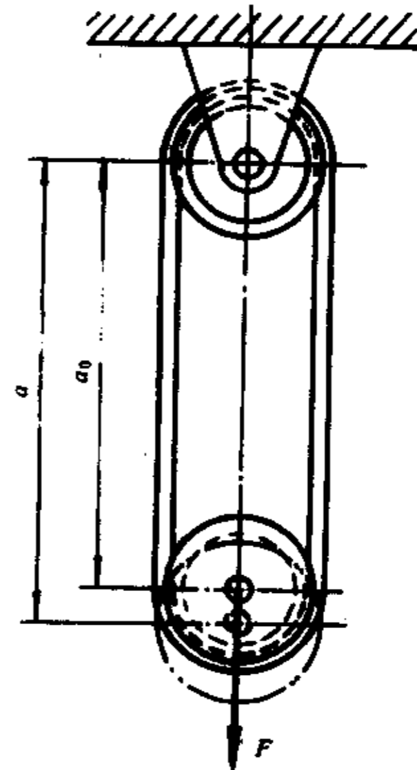
图 2 疲劳试验机
