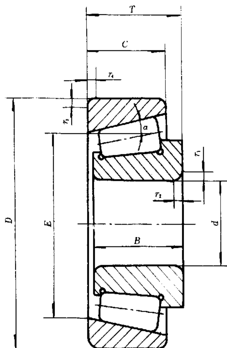
圆锥滚子轴承 30000 型
