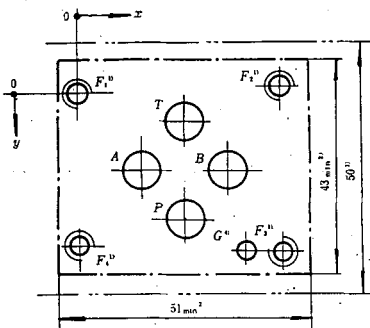
图 2 主油口最大直径为 6.3mm 的压力控制阀、顺序阀、 卸荷阀、节流阀和单向阀的安装面(代号:03)
