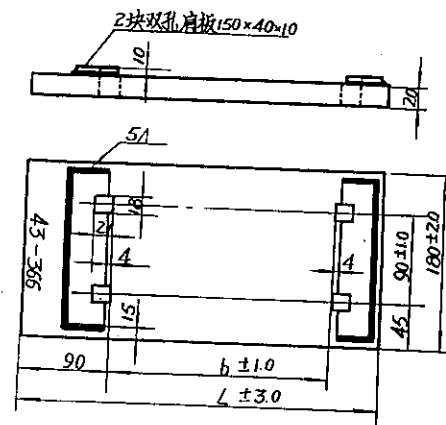
每米43公斤钢轨护轨平肩垫板
